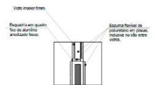
Detalhe 01 Escala 1/50
