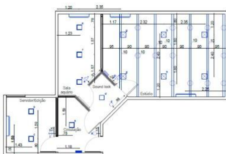
Esquema luminotécnico/ ar condicionado Escala 1/50
