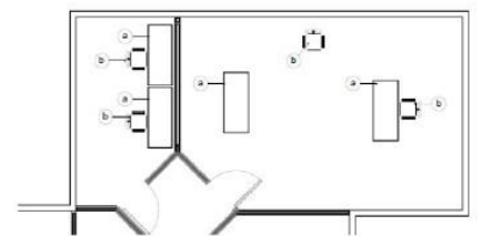
Planta Baixa - Layout Escala 1/100
