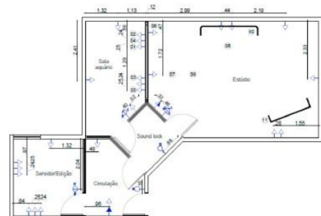
Esquema elétrico Escala 1/50
