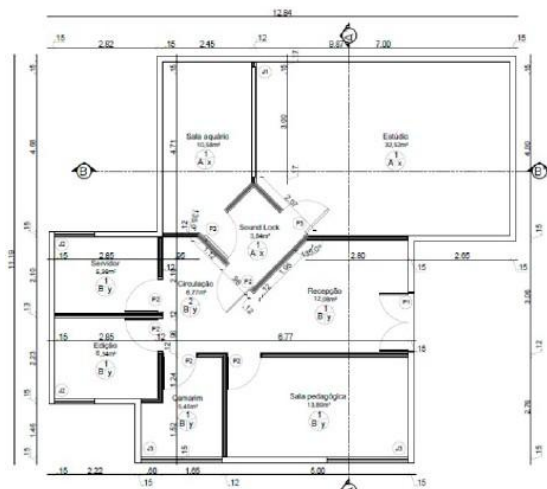
Planta Baixa - Especificações Escala 1/100
