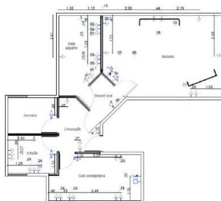
Esquema elétrico Escala 1/65
