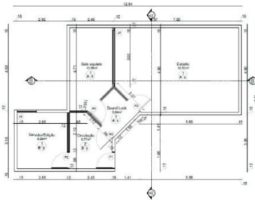
Planta Baixa - Especificações Escala 1/100
