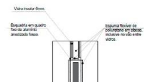
Detalhe 01 Escala 1/100
