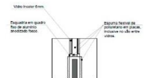
Detalhe 01 Escala 1/10
