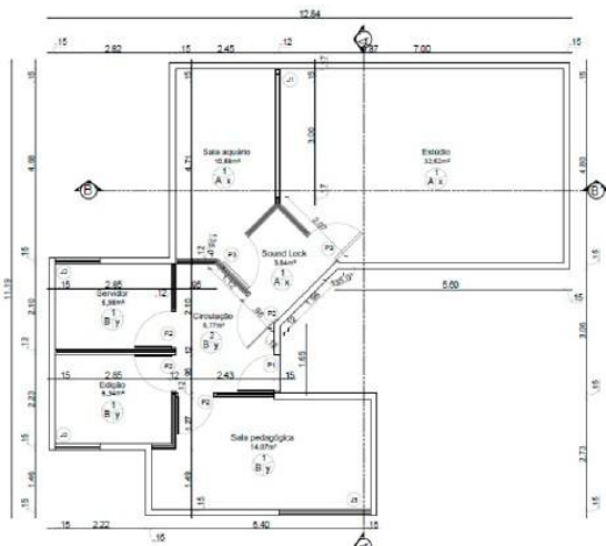
Planta Baixa - Especificações Escala 1/50
